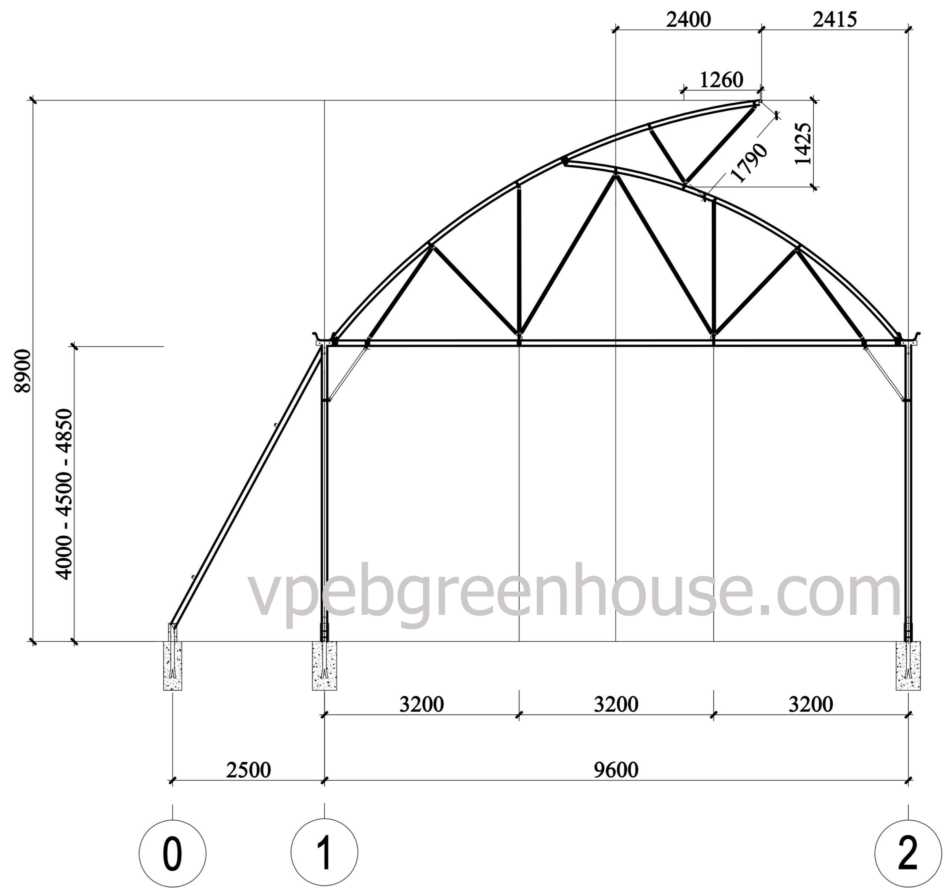
MẶT CẮT KÈO TRUNG GIAN
