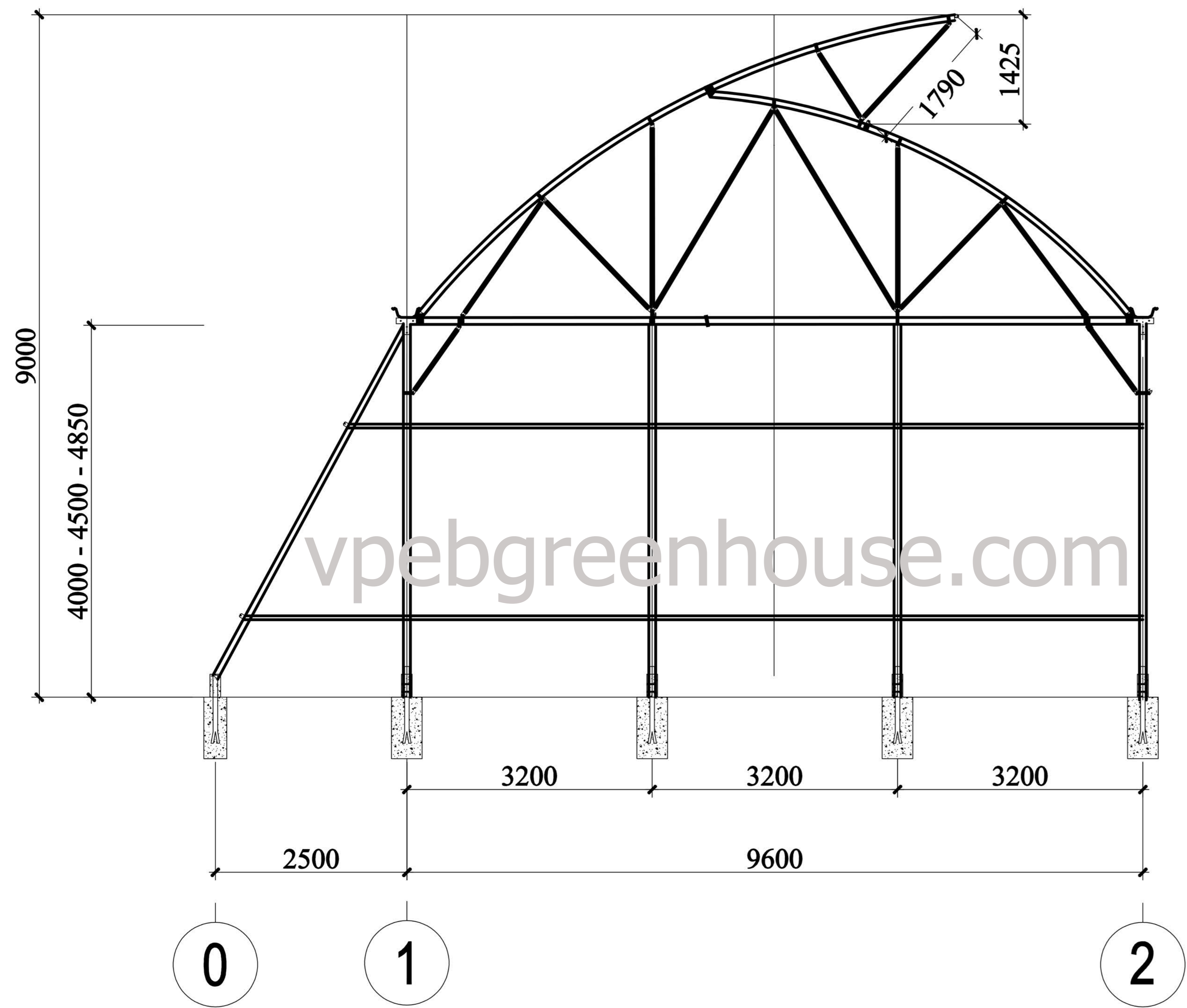
MẶT CẮT KÈO ĐẦU HỒI
