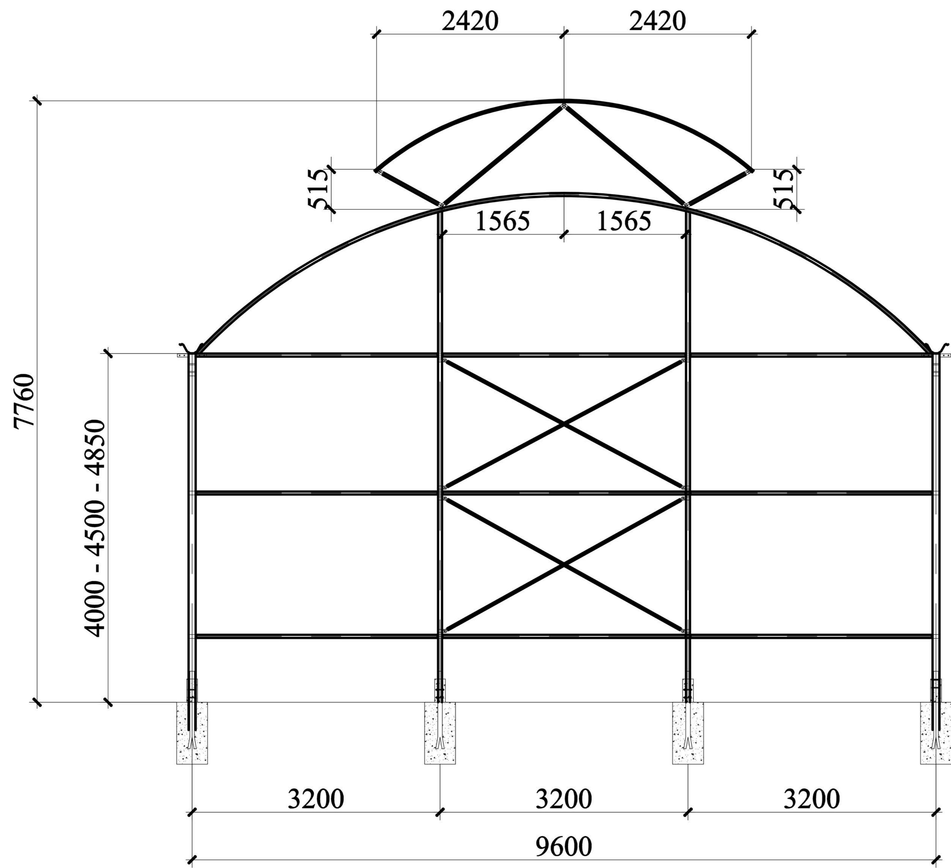
MẶT CẮT CHI TIẾT KÈO ĐẦU HỜI
